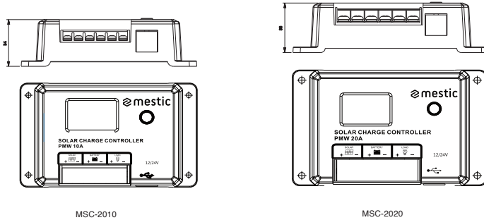
MSC-2010
